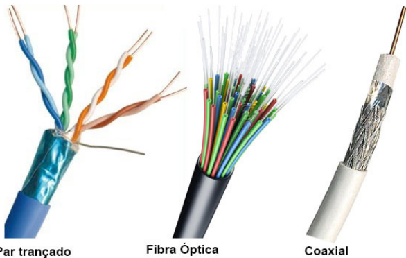
Fonte: http://eletronicaapolo.com.br/novidades/o-que-e-o-cabo-de-rede-par-trancado
