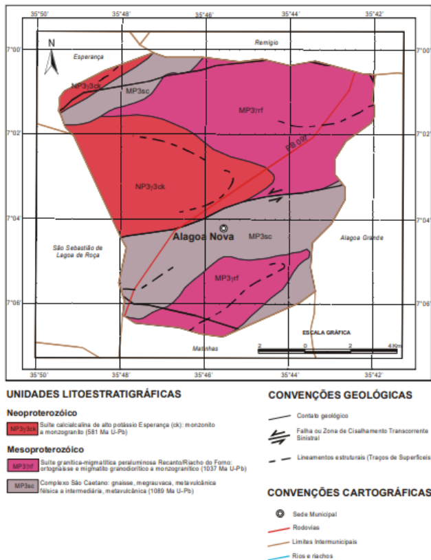
Figura 3 – Mapa Geológico
