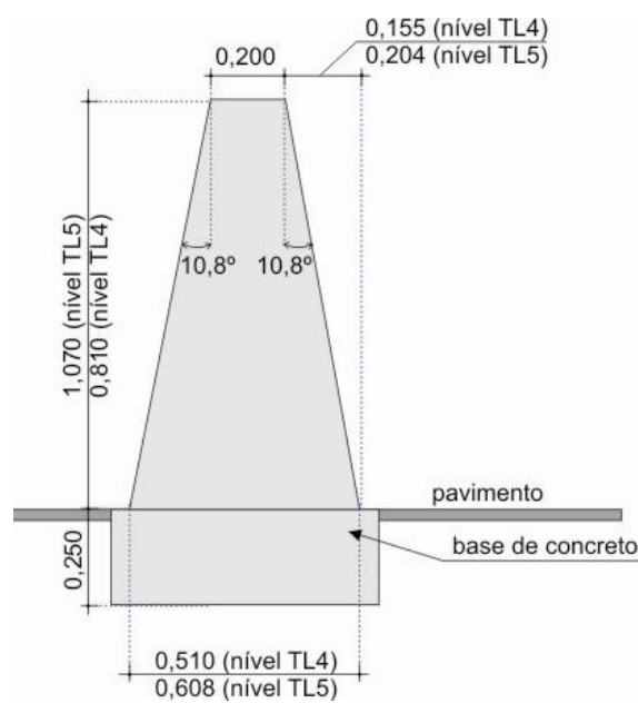
Barreira “Texas” dupla
