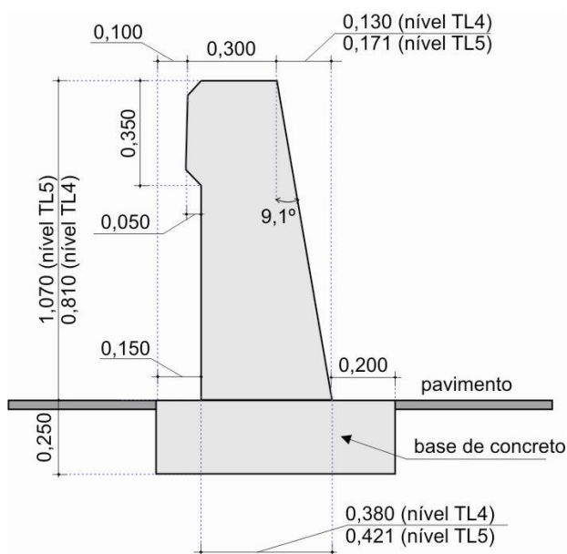
Barreira “Califórnia” simples
