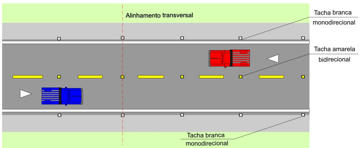
Alinhamento transversal das tachas Figura 4.34
