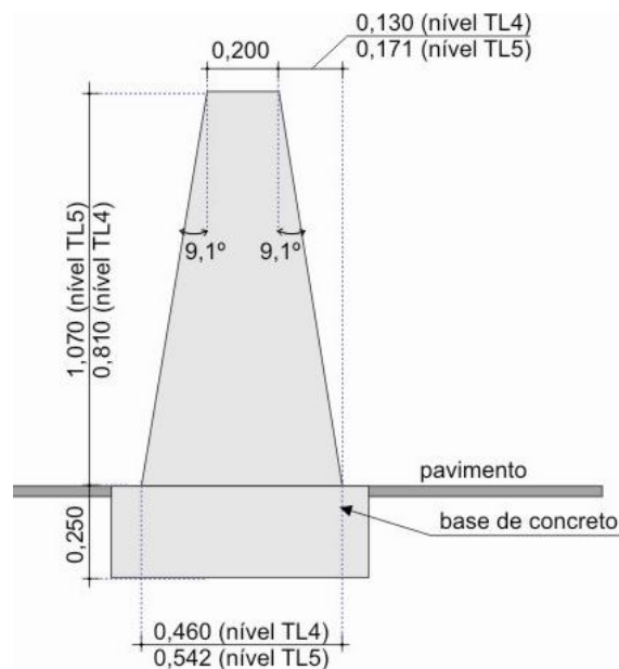
Barreira “Califórnia” dupla
