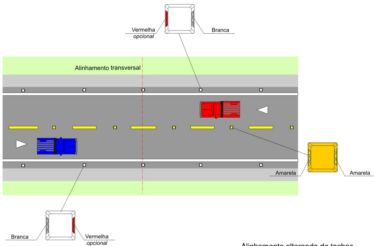
Alinhamento alternado de tachas Figura 4.35
